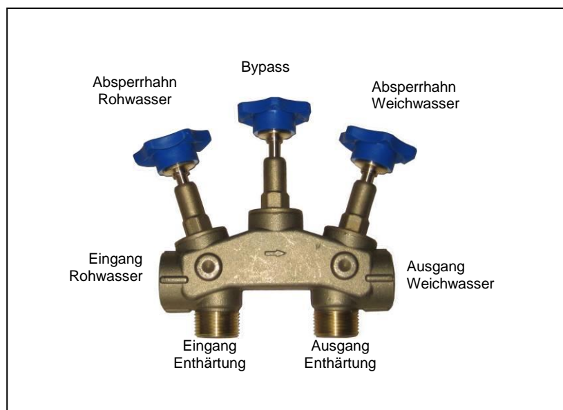
Abbildung 4: Montageblock
