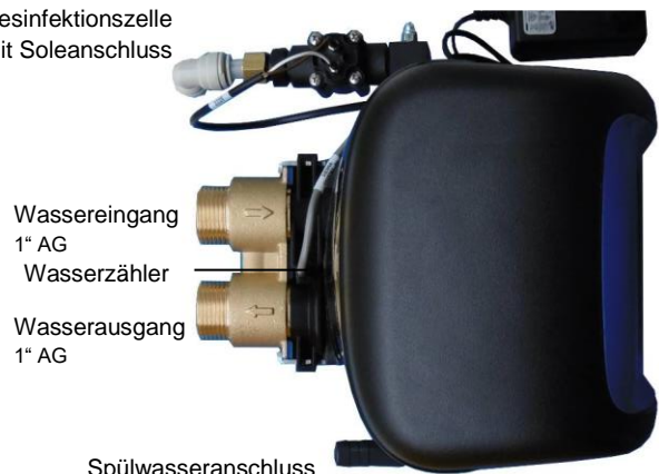
Spülwasseranschluss
